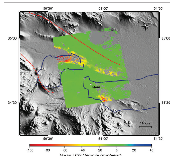
شکل ۳- میدان سرعت متوسط حاصل از پردازش تصاویر Sentinel مربوط به دشت‌های جعفرآباد و قنات بعد از حذف خطاها. کادر سیاه معرف منطقه‌ای بوده که به عنوان مرجع در نظر گرفته شده است. مثلث سفید موقعیت شهر قم را نشان می‌دهد. محدوده‌هایی که با رنگ آبی مشخص شده‌اند محدوده دشت‌ها در استان قم هستند.
